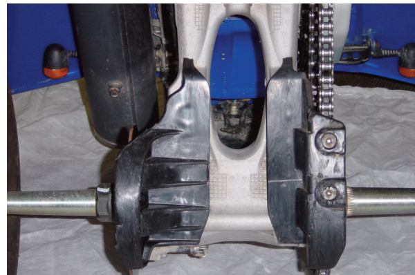
Figura 2 - Paracatena inferiore
