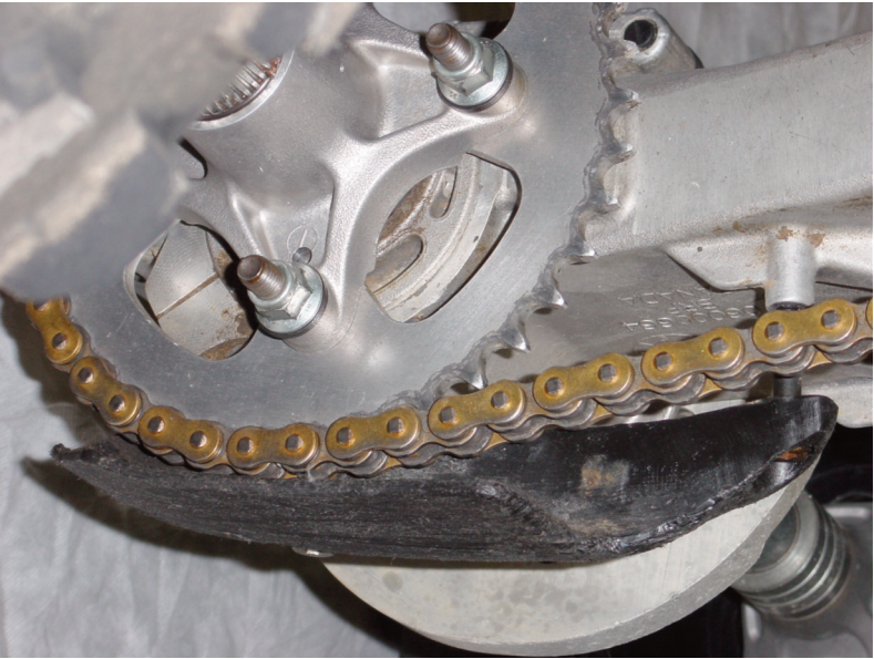
Figura 3 - Paracatena inferiore
